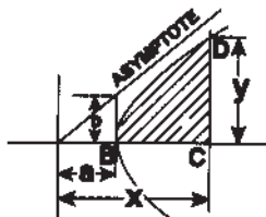
Hyperbola
